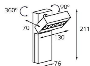
LED модуль 220V 5x2W 3000K 850 lm 46° IP20 DIM Дополнительно: возможна замена внешней панели (арт. Cover Focus white/ black/ alu/ gold)
